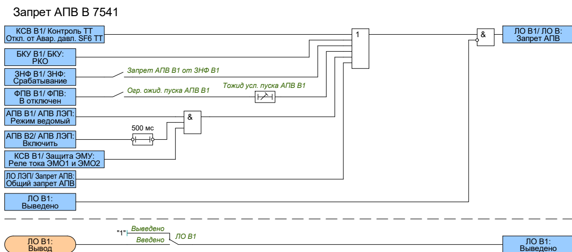
Рисунок 2.69 – Функциональная схема запрета АПВ В1
