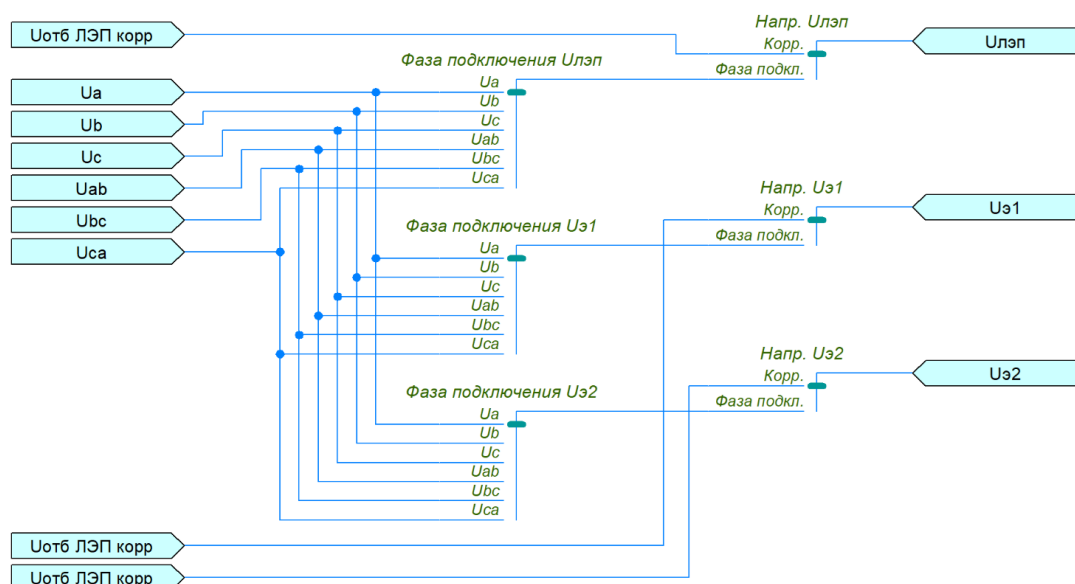
Рисунок 2.84 – Функциональная схема настройки аналоговых значений U_{лэп} , U_{э1} , U_{э2}
