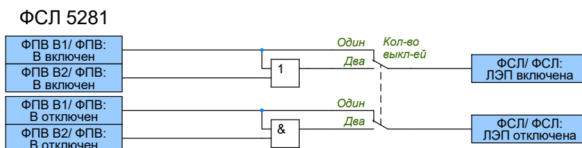
Рисунок 2.82 – Функциональная схема логики ФСЛ
