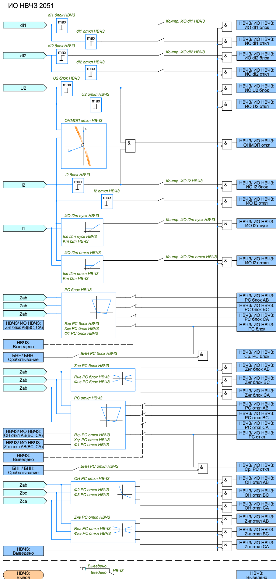
Рисунок 2.9 – Измерительные органы НВЧ3
