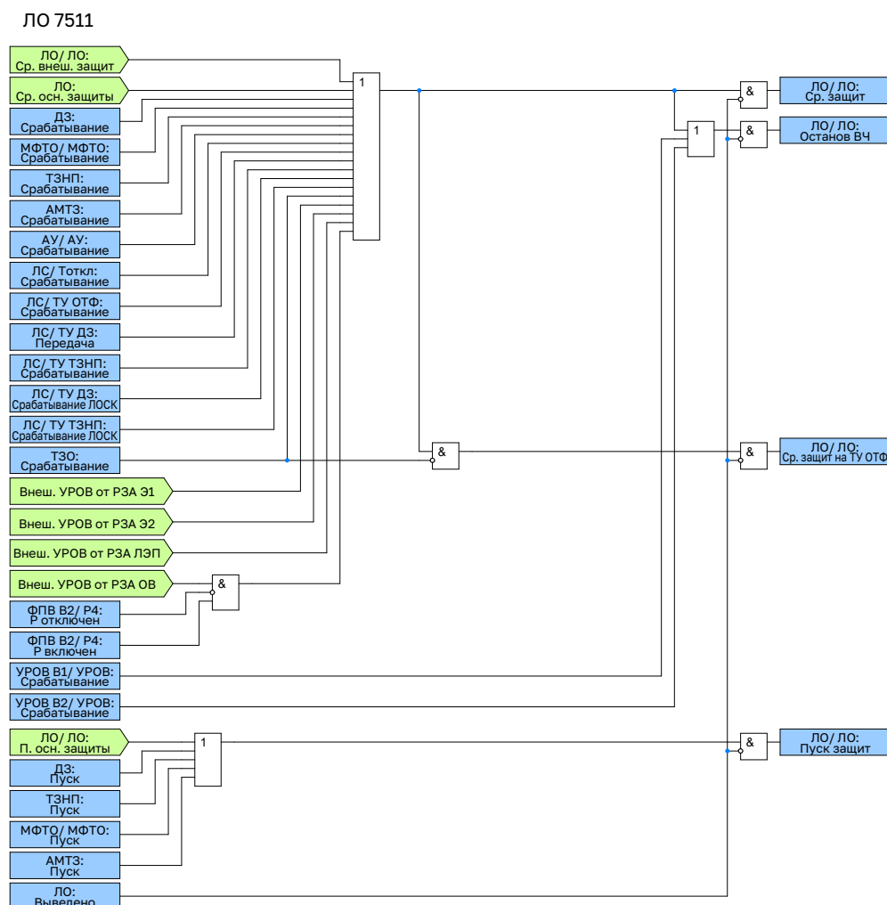
Рисунок 2.77 – Функциональная схема общей логики отключения
